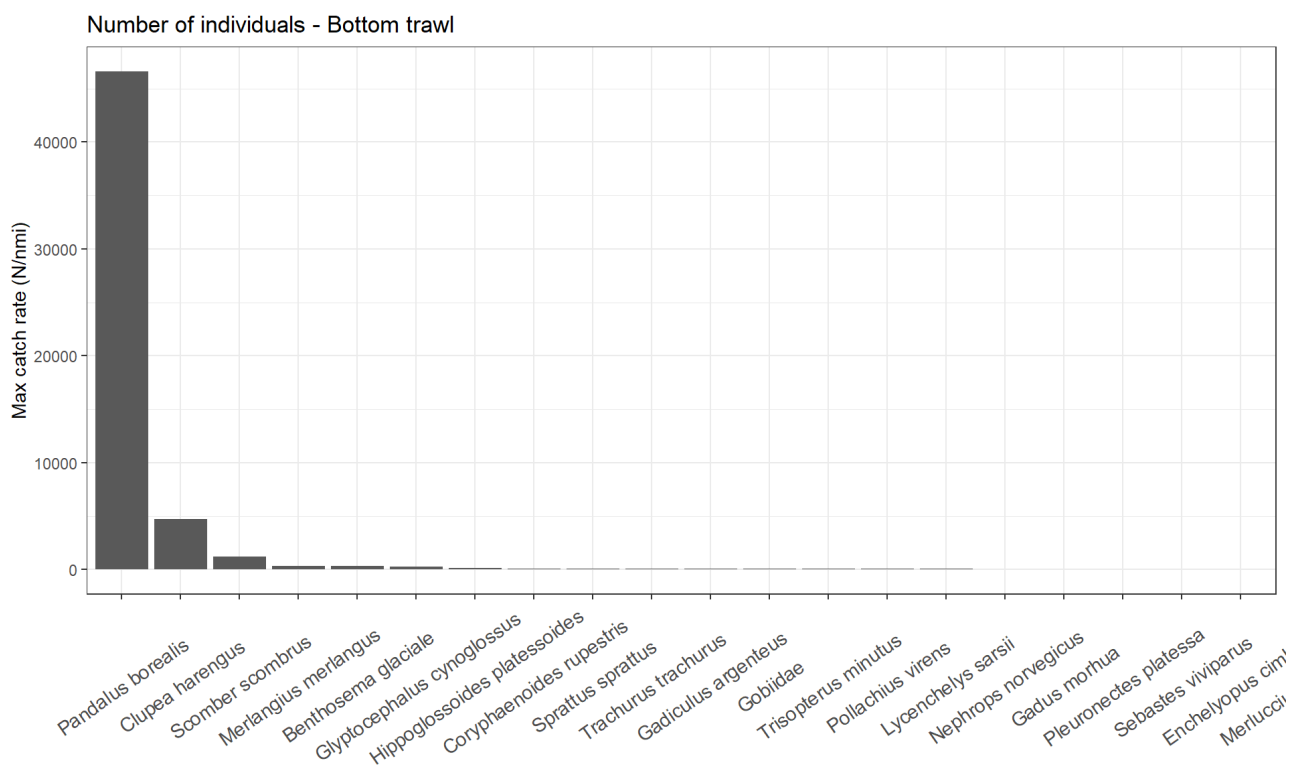
Figur 6.5: De 20 mest vanlige artene rangert etter den høyeste fangstraten i antall individer (antall/nm) i fangstene på reketoktet i 2021. Se Vedlegg 4 for norske, engelske og latinske navn på alle artene på toktet.
