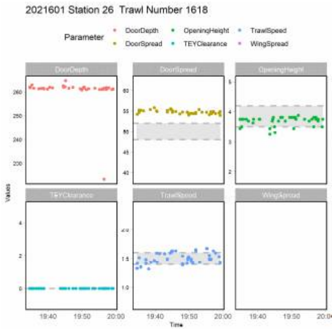
Figur 10.1: Scanmar-data fra trålstasjon 26: dørdepth (m), dørspredning (m), trållåpning (m), trålløye klaring (m), trållfart (m/s) and vingespredning (m) (ikke logget for dette halet). Skraverte felt viser tidligere tillatte intervall for sjøtestingshal for dørspredning (48–52 m), trållåpning (3,5–4,2 m) og trållfart (1,4–1,6 m/s).
