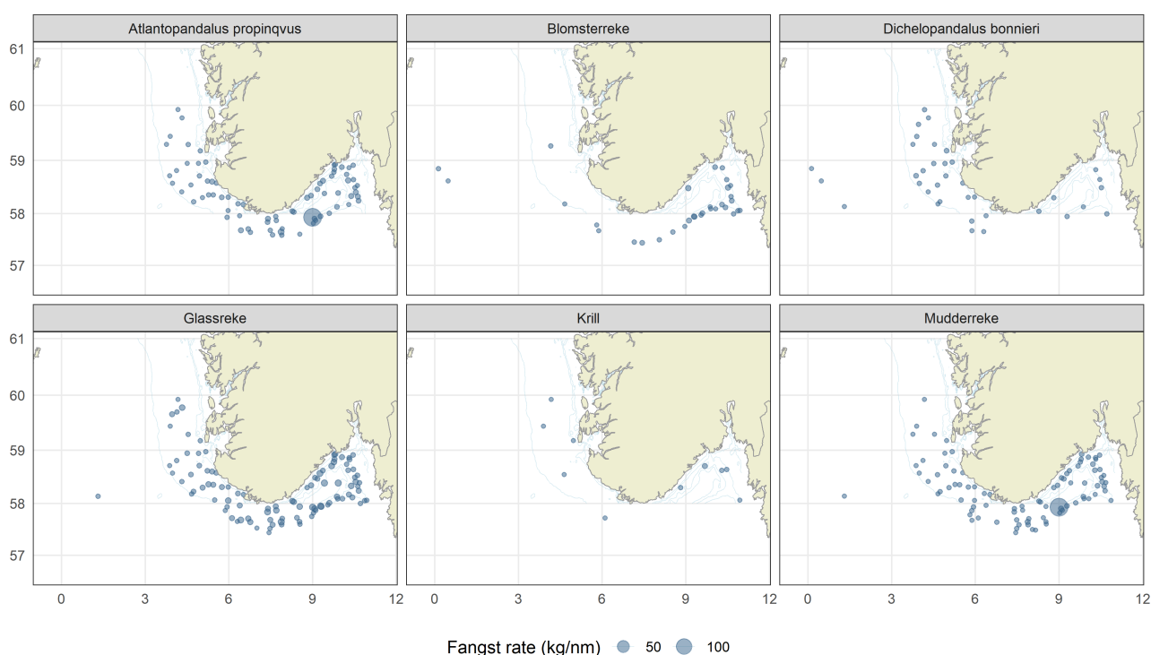
Figur 6.20: Fordeling av Atlantopandalus propinqus , Pandalus montagui (blomsterreke), Dichelopandalus bonnieri , Pasiphea spp (glassreker), Euphausiacea (krill) og Pontophilus spp (mudderreker) på reketoktet i 2021. Størrelsen på boblene er proporsjonal med fangstraten (kg/nm).
