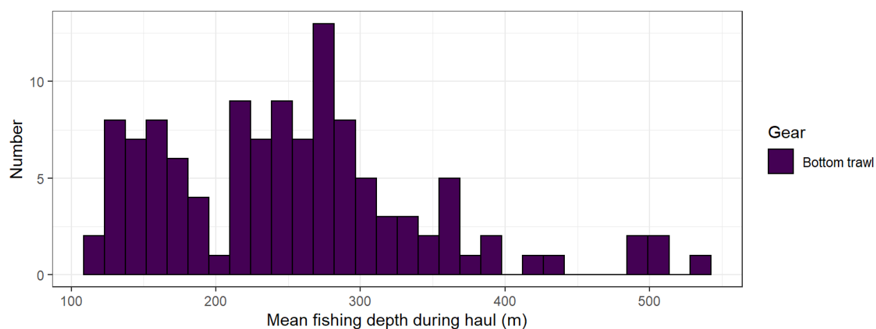
Figur 6.2: Histogram av gjennomsnittlig fiskedyp på 116 av totalt 121 bunntrålstasjoner på reketoktet i 2021 (faste stasjoner, to stasjoner fra rekefisker og stasjoner på Fladengrunn). Det manglet fiskedyp for enten start- eller sluttposisjon på fem trålstasjoner.
