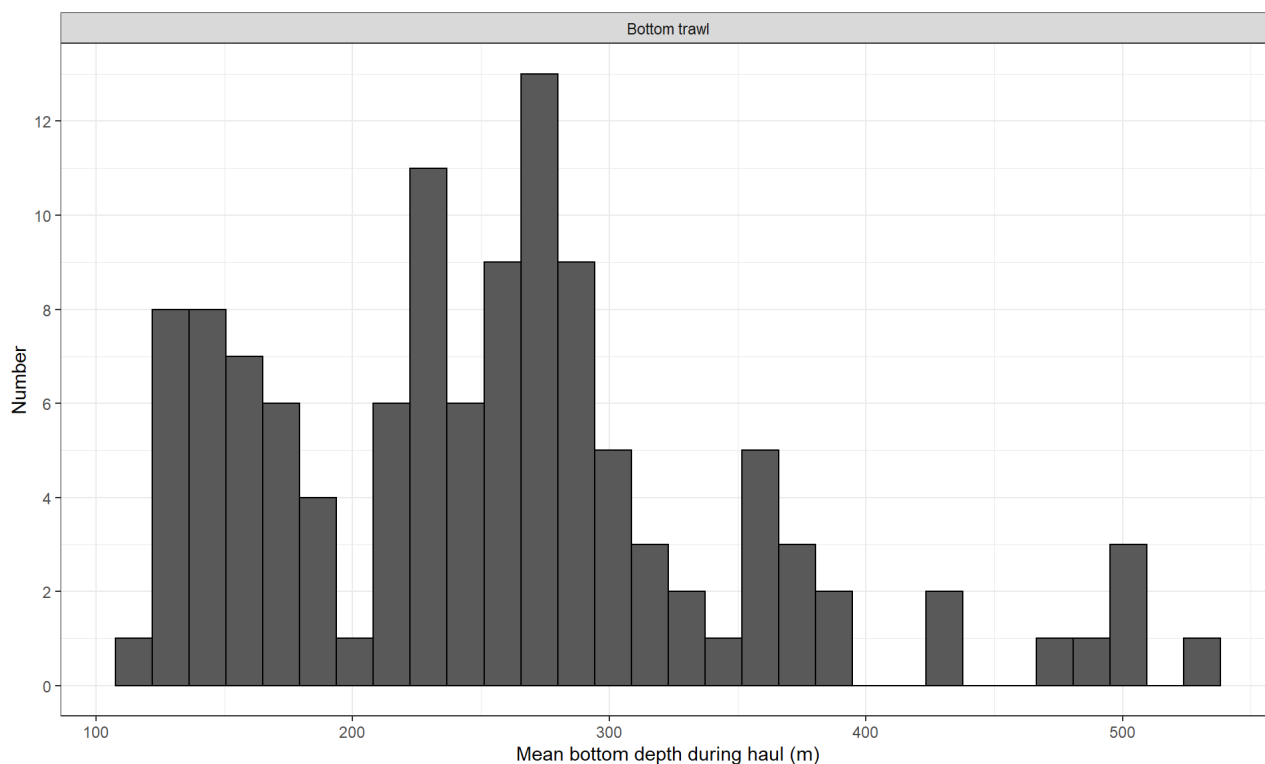
Figur 6.1: Histogram av gjennomsnittlig bunndyp på 118 av totalt 121 bunntrålstasjoner på reketoktet i 2021 (faste stasjoner, to stasjoner fra rekefisker og stasjoner på Fladengrunn). Det manglet bunndyp for sluttposisjon på tre trålstasjoner.
