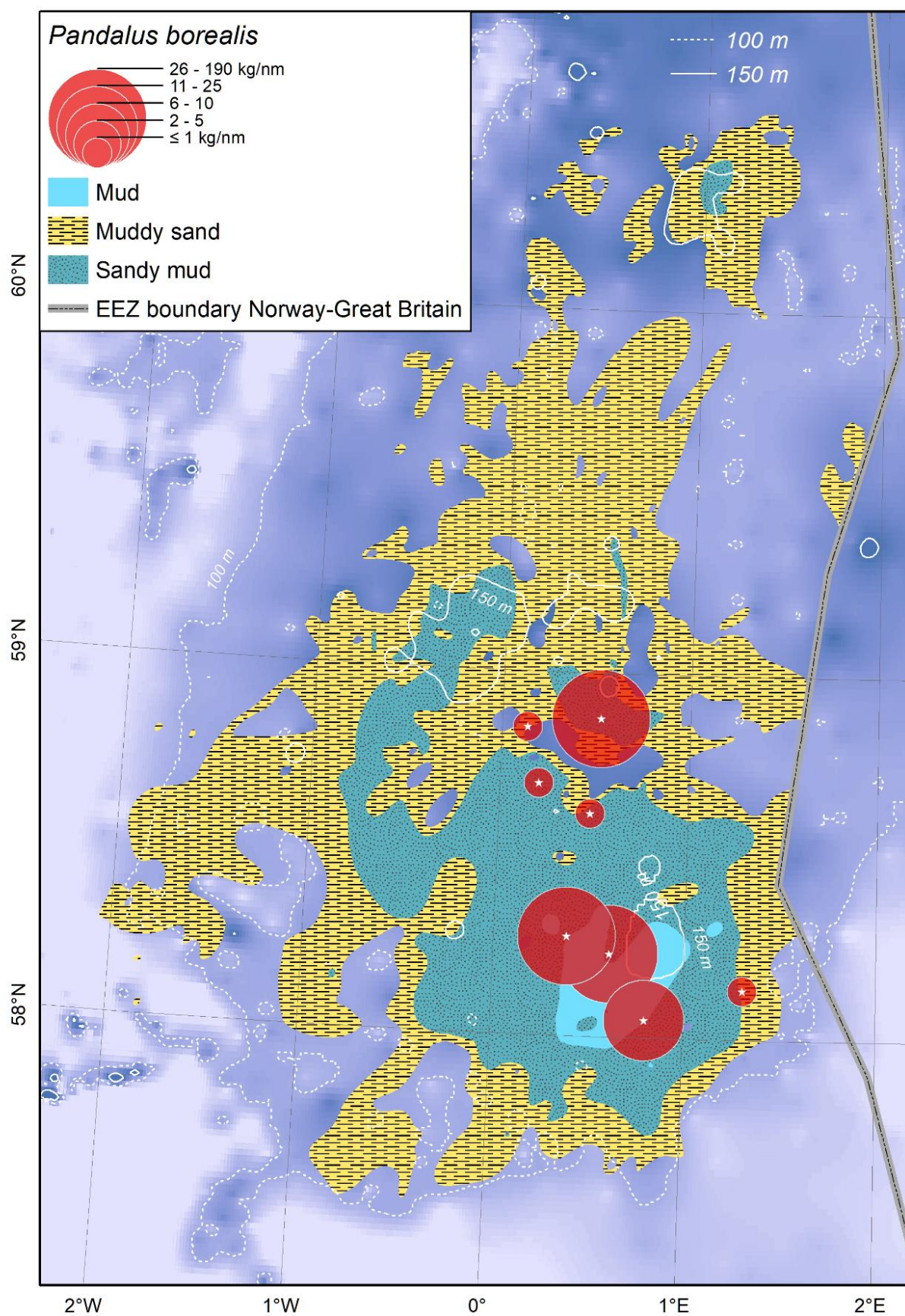
Figur 6.10: Fordeling av dypvannsreke på reketoktet i 2021 på Fladengrunn. Boblestørrelsen er proporsjonal med fangstraten.
