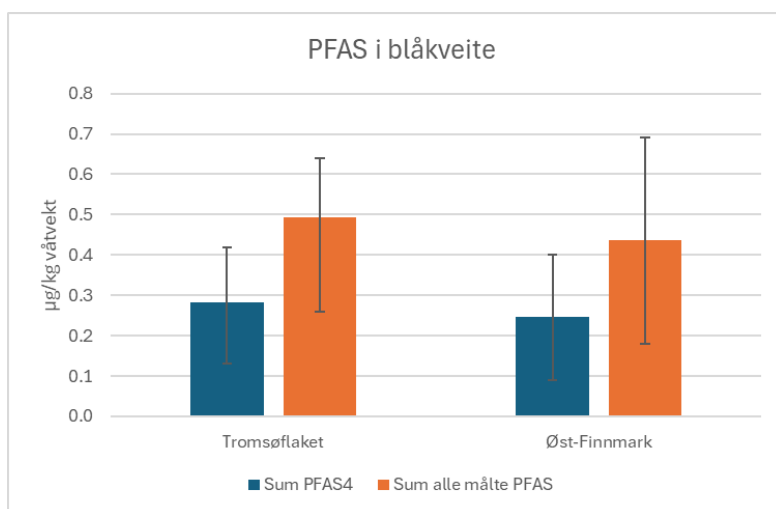
Figur 5. Konsentrasjon av Sum PFAS4 (Lower bound (LB) summen av PFOS, PFOA, PFHxS og PFNA) og sum alle målte PFAS i blåveite, prøvetatt i ulike områder. Grenseverdien for sum PFAS4 som gjelder for de fleste fiskearter er 2,0 µg/kg.
