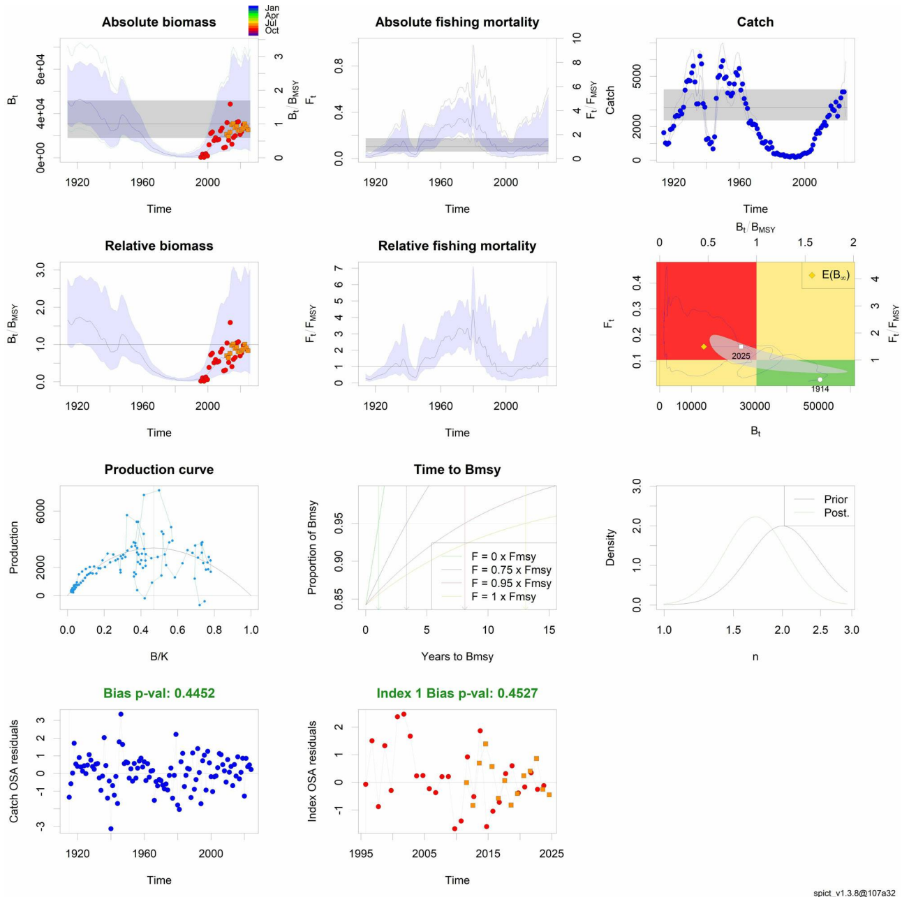
Figur 4: Kveite i norsk økonomisk sone nord for 62°N, ICES-område 1-2. SPiCT-output fra den endelige bestandsmodellen. Standardfigurer fra SPiCT som viser absolutte og relative bestandstrender, produksjonskurven og residualer til input-tidsseriene.
