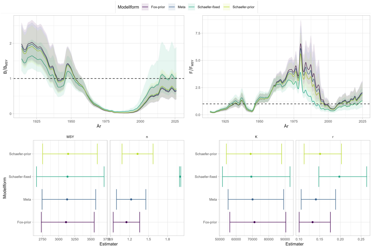
Figur 16: Kveite i norsk økonomisk sone nord for 62°N, ICES-område 1-2. SPiCT-estimer ved ulike verdier av modellform-prior n : prior basert på Fox-modell (gjennomsnitt = 1, standardavvik = 0,5) og på en metastudie (1,478, 0,6), fiksert til Schaefer-modell (2, 0), og en mindre informativ Schaefer-prior (2, 0,5). Figuren viser B/B_{MSY} , F/F_{MSY} , MSY , n , bæreevne K og bestandsvekst r . Linjer og punkter tilsvarer estimert gjennomsnitt, fargelagte områder og feillinjer angir 95% konfidensintervaller.
