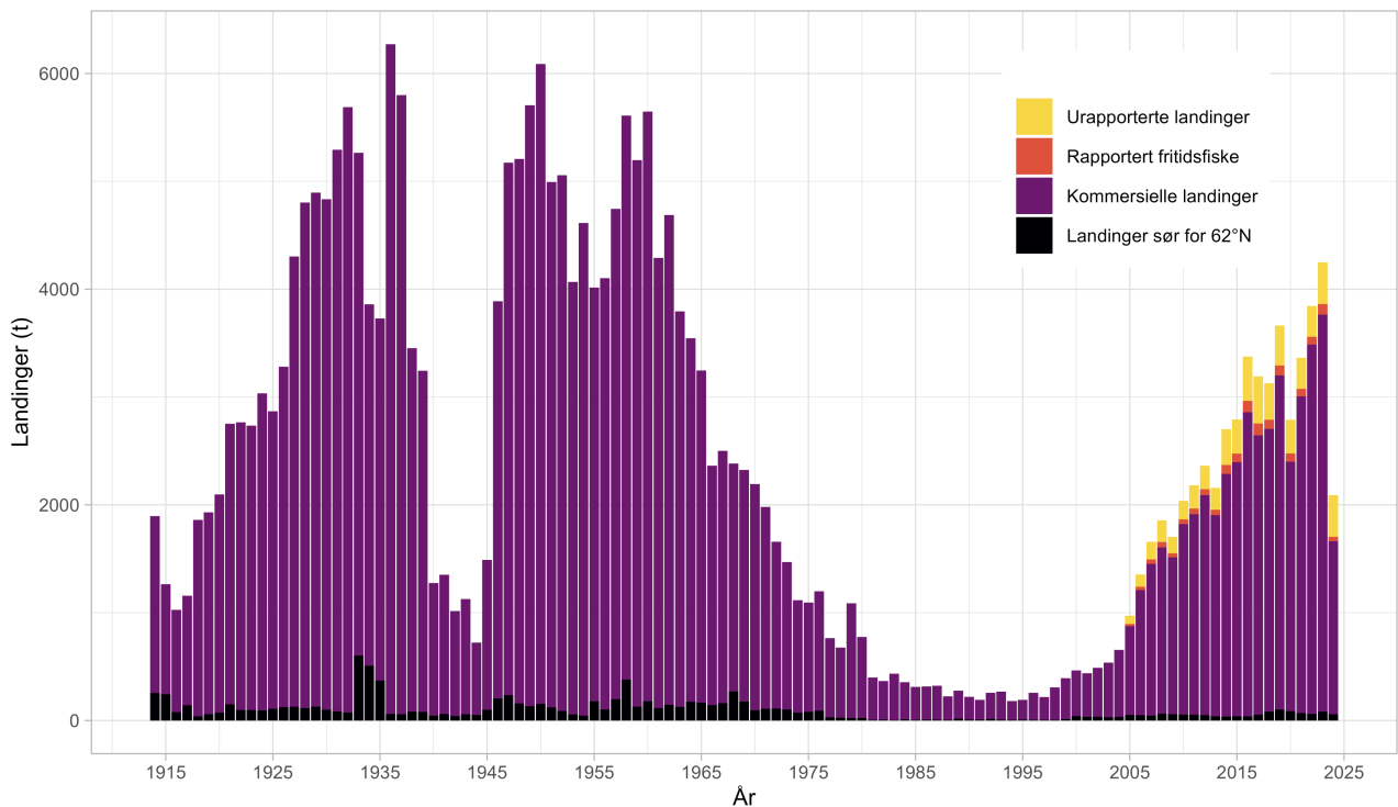
Figur 1: Kveite i norsk økonomisk sone, ICES-områder 1-4. Tidsserie av rapporterte landinger (lilla), rapporterte landinger av fritidsfisker (rød), antatt urrapporterte landinger av fritidsfisker (gul) nord for 62°N, og rapporterte landinger sør for 62°N (sort). Landinger i 2024 er kun tom. juli.
