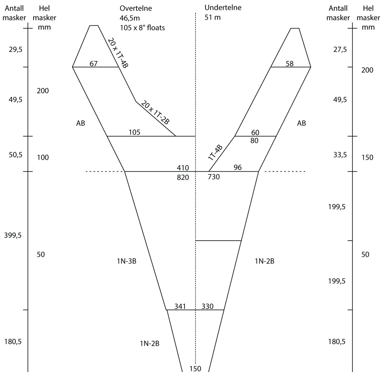
Figur 12. Skjematisk tegning av Skjervøytrål.
